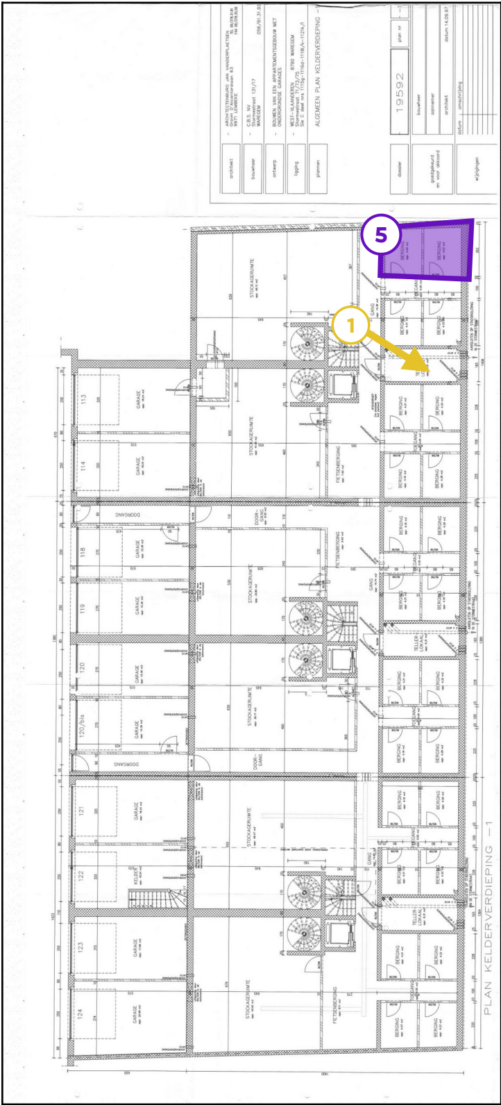
Legende van plan 1.3: Stormestraat 71-73-75 Algemeen plan kelderverdiepi
